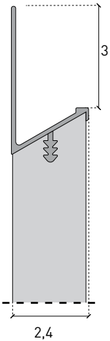
Sezione anta Door section
